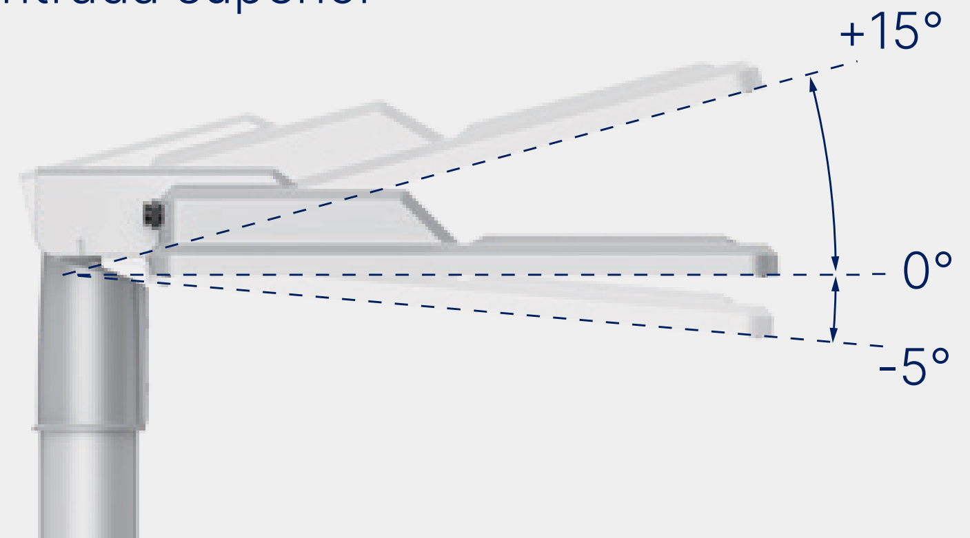
Entrada superior
