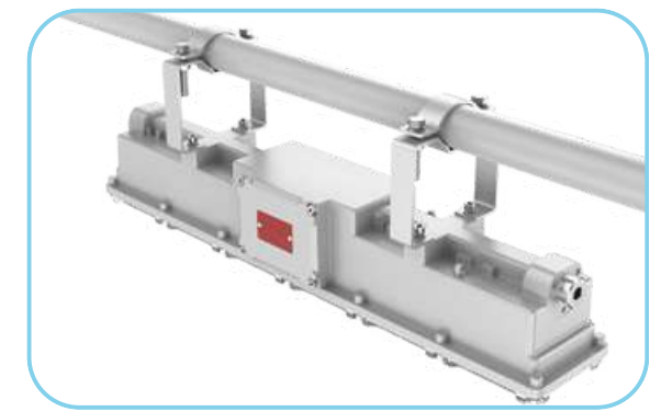
Montaje colgante
